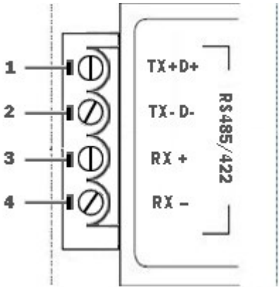
端子接口管脚定义
